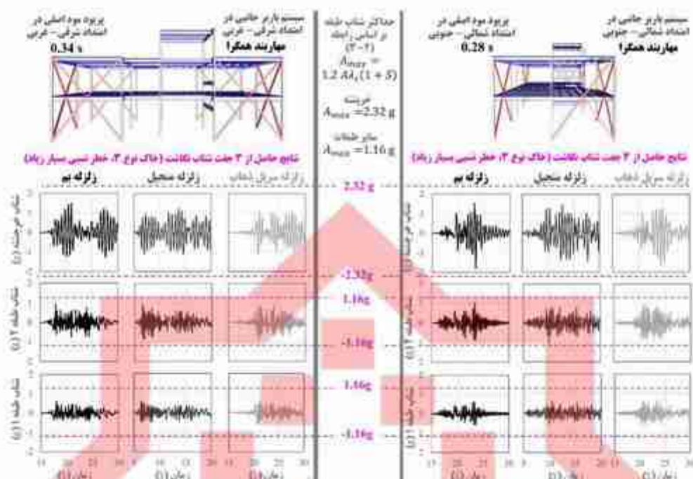
شکل پ-۵-۱ بررسی دقت رابطه (۲-۳) در تخمین حداکثر شتاب لرزه‌ای خارج از صفحه وارد بر دیوار برای یک ساختمان ۳ طبقه فولادی ساخته شده در منطقه‌ای با خاک نوع ۳ و خطر لرزه‌ای نسی بسیار زیاد.
