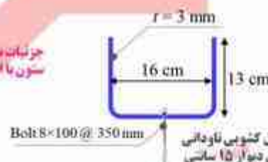
شکل پ-۵-۱۹ جزئیات نهایی اتصال دیوار به ستون به صورت ناودانی سرنسری
