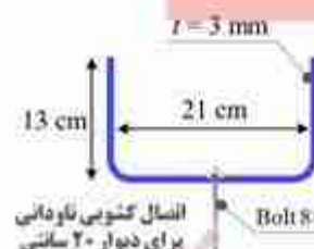
شکل پ-۵-۱۹ جزئیات نهایی اتصال دیوار به ستون به صورت ناودانی سرنسری
