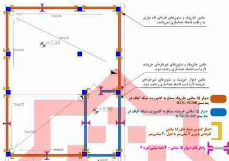
شکل پ-۱۰- تیب بندی دیوارها، جانمایی و اداری های قائم و اتصالات کنونی در بام و خرپشته
