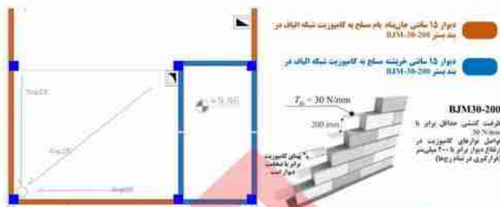
شکل پ-۴-۶: تیپ بندی دیوارهای جان پناه بام و خریشته (ستون‌ها به اندازه ارتفاع جان پناه از کف بام امتداد یافته است. در محل خریشته، ستون‌ها تا سقف خریشته امتداد دارند.)
