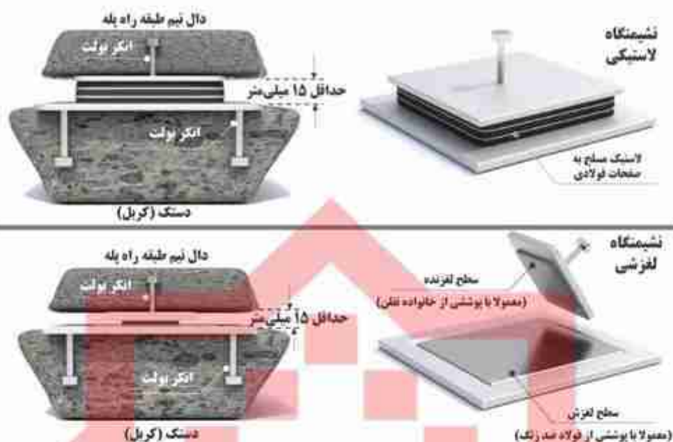
شکل ۴-۳۷ نمونه‌ای از جزئیات نشیمنگاه‌های لاستیکی و لغزنی به منظور جداسازی راه پله
