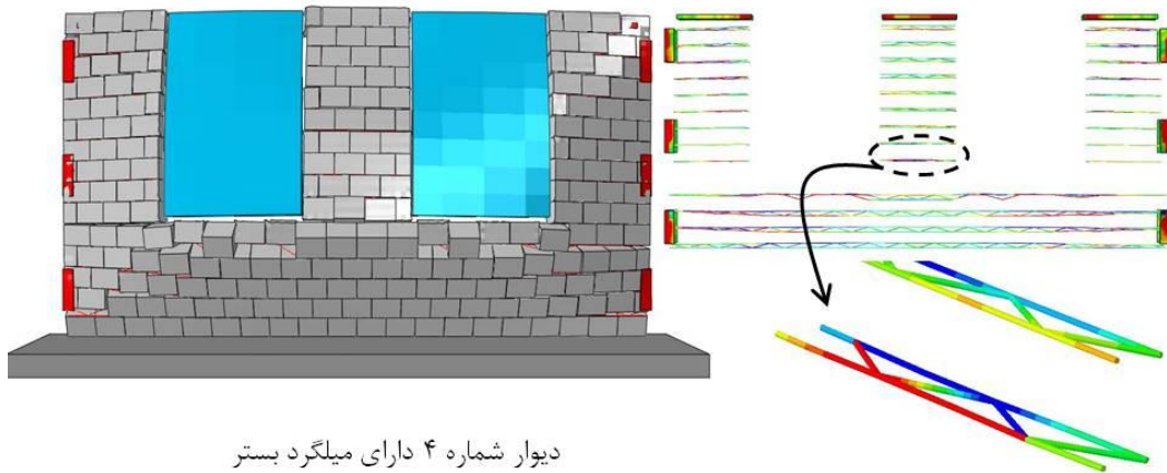
شکل ۱۱-۱۵. نحوه فروریزش دیوار شماره ۴ با و بدون میلگرد بستر (به منظور نمایش بهتر ترک ها در تغییر شکل دیوار بزرگنمایی شده است لذا در برخی لبه ها اتصالات در شکل مشخص نیستند)
