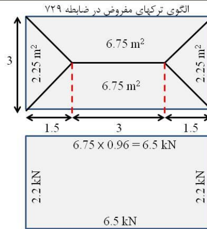
شکل ۱۱-۳. شبیه سازی دیوار شماره ۱ در حالتی که فاقد میلگرد بستر باشد
