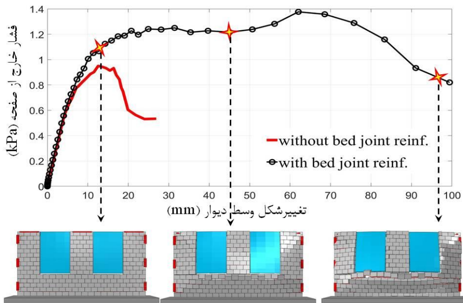
شکل ۱۱-۱۶. مقایسه رفتار خارج از صفحه دیوار شماره ۴ با و بدون میلگرد بستر-منحنی ها smooth شده اند.
