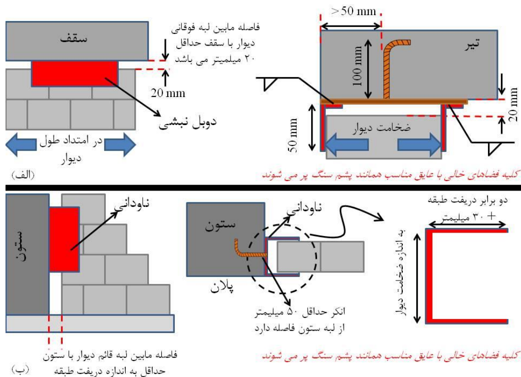
شکل ۸-۱. نمونه ای از اتصالات کشویی (الف) دیوار به سقف و (ب) دیوار به ستون
