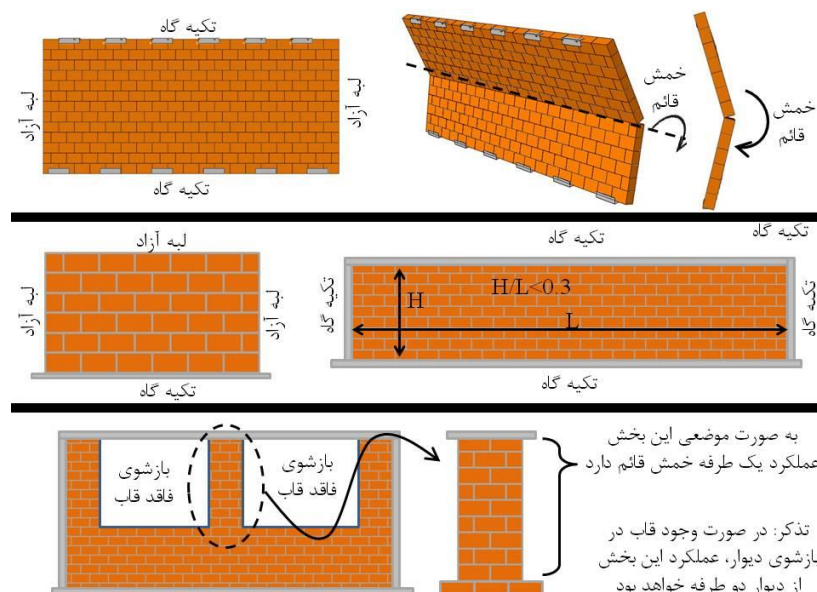
شکل ۳-۱. نمونه هایی از دیوارهای بنایی با عملکرد یک طرفه خمش قائم
