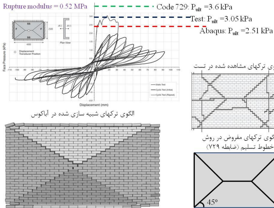
شکل ۱۰-۴. ظرفیت دیوار شماره ۱ از سه روش آزمایشگاهی، مدل المان محدود و ضابطه ۷۲۹ (بدون ضریب کاهش مقاومت).
