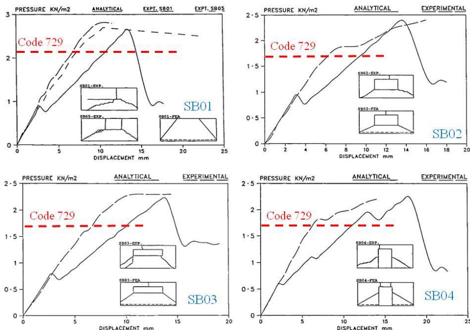
شکل ۱۰-۹. رفتار چهار نمونه از دیوارهای تست شده به همراه تخمین ضابطه ۷۲۹ از مقاومت نهایی آنها (خطوط توپر نتایج آزمایشگاهی می باشند).
