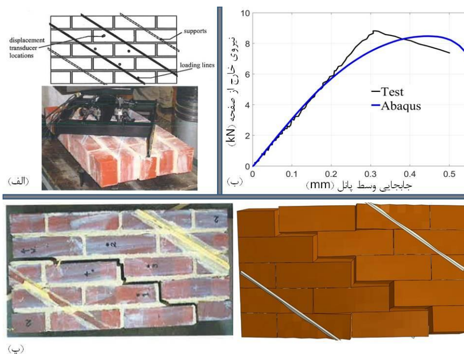
شکل ۱۰-۲. صحت سنجی مدل آباکوس دیوار در خمش مورب (الف) چیدمان تست Willis (2004). (ب) مقایسه منحنی نیرو-تغییر مکان اندازه گیری شده در تست و شبیه سازی شده در آباکوس. (پ). الگوی ترکهای مشاهده شده در تست و مدل آباکوس
