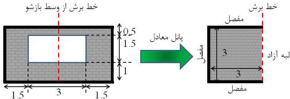
شکل ۶-۱۱. ساخت پانل معادل دیوار شماره ۲
