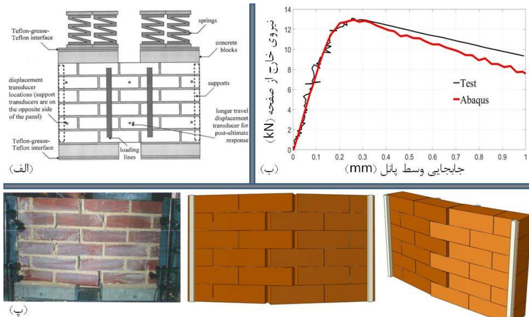
شکل ۱۰-۱. صحت سنجی مدل آباکوس دیوار در خمش افقی (الف) چیدمان تست Willis (2004). (ب) مقایسه منحنی نیرو-تغییر مکان اندازه گیری شده در تست و شبیه سازی شده در آباکوس. (پ). الگوی ترکهای مشاهده شده در تست و مدل آباکوس
