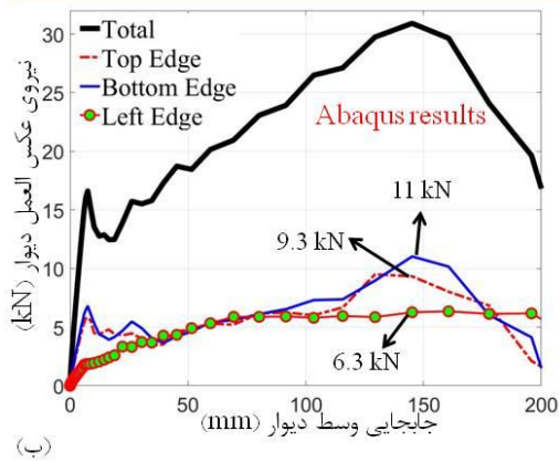
شکل ۱۱-۴. شبیه سازی دیوار شماره ۱ در حالتی که دیوار مسلح به میلگرد بستر باشد (مطابق طراحی انجام شده در این بخش)
